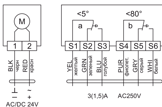
Рисунок 6.2 – Схемы подключения приводов RLF
