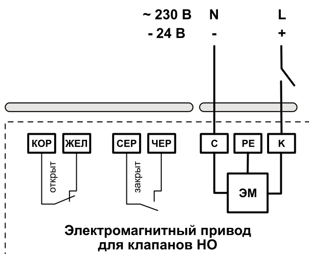
Рисунок 6.4 – Схемы подключения приводов ЭМП
