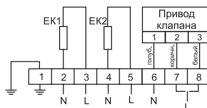
(P-Ik/220)/-60°C
