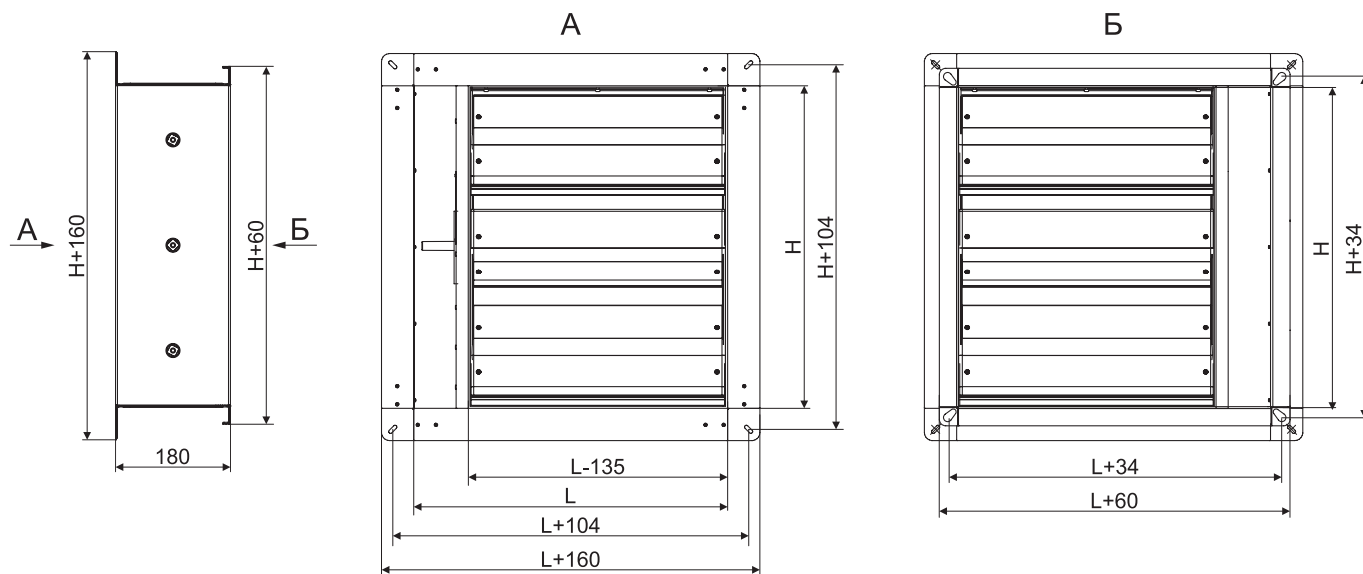
Стеновой тип
