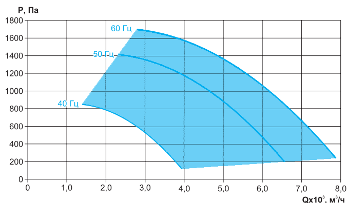
VCB-LT-630-O/35-РЦ-3,0/3000/220-380-Y2
