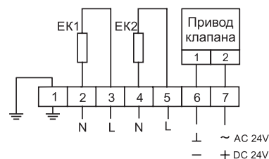
(М-1к/24)/-40°С (М-1к/24)/-60°С
