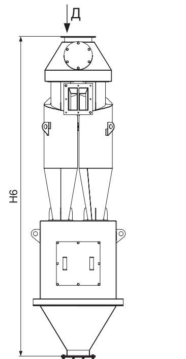
ЦН-15-2СП
