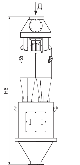
ЦН-11-2СП
