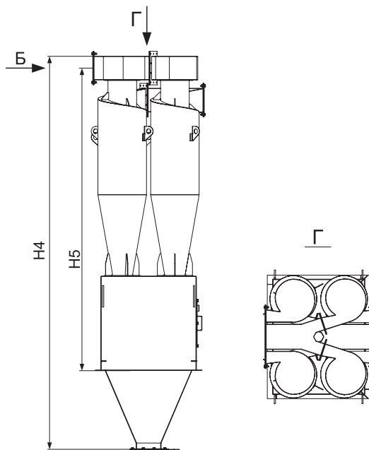
ЦН-11-4УП
