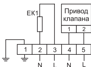
(М-1к/220)/-20°С
